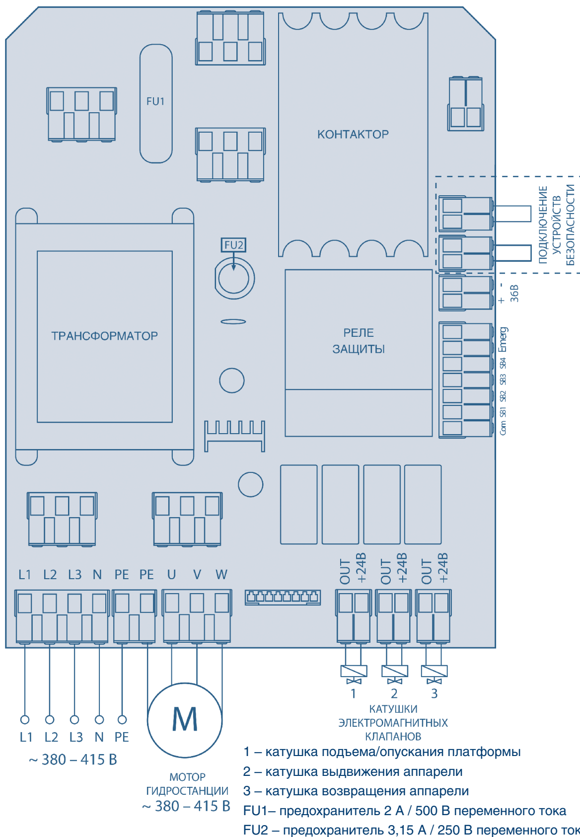
Рис. 5.1. Общая схема электрических подключений
