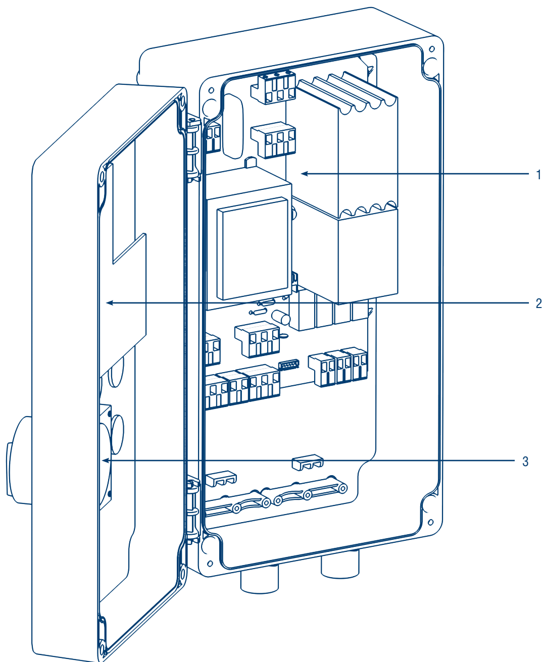
Рис. 2.1. Конструкция блока управления
