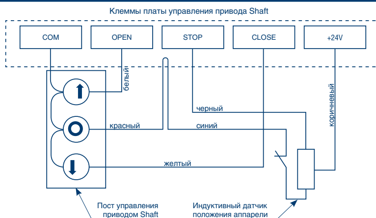
Рис. 5.2. Схема подключения индуктивного датчика положения аппарата*
