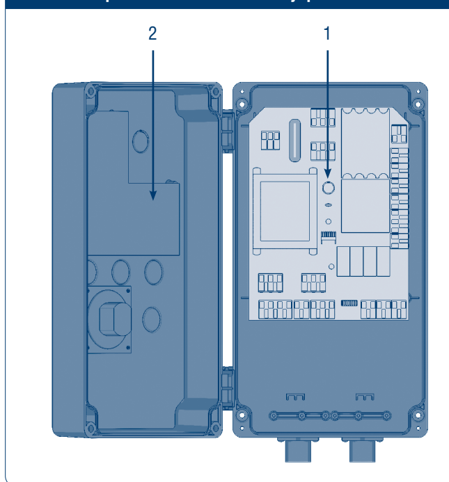
Рис. 3.2. Открытое положение блока управления
