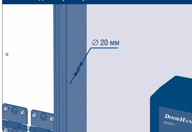
Рис. 1.1.1. Диаметр отверстия
